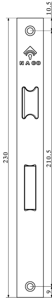
Right view Scale: 1:1
